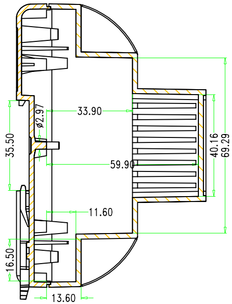
SEC A-A
