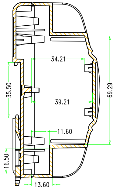
SEC A-A
