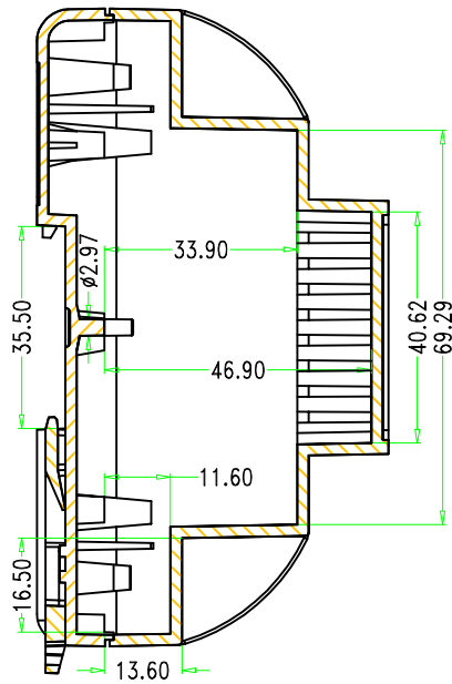
SEC A-A
