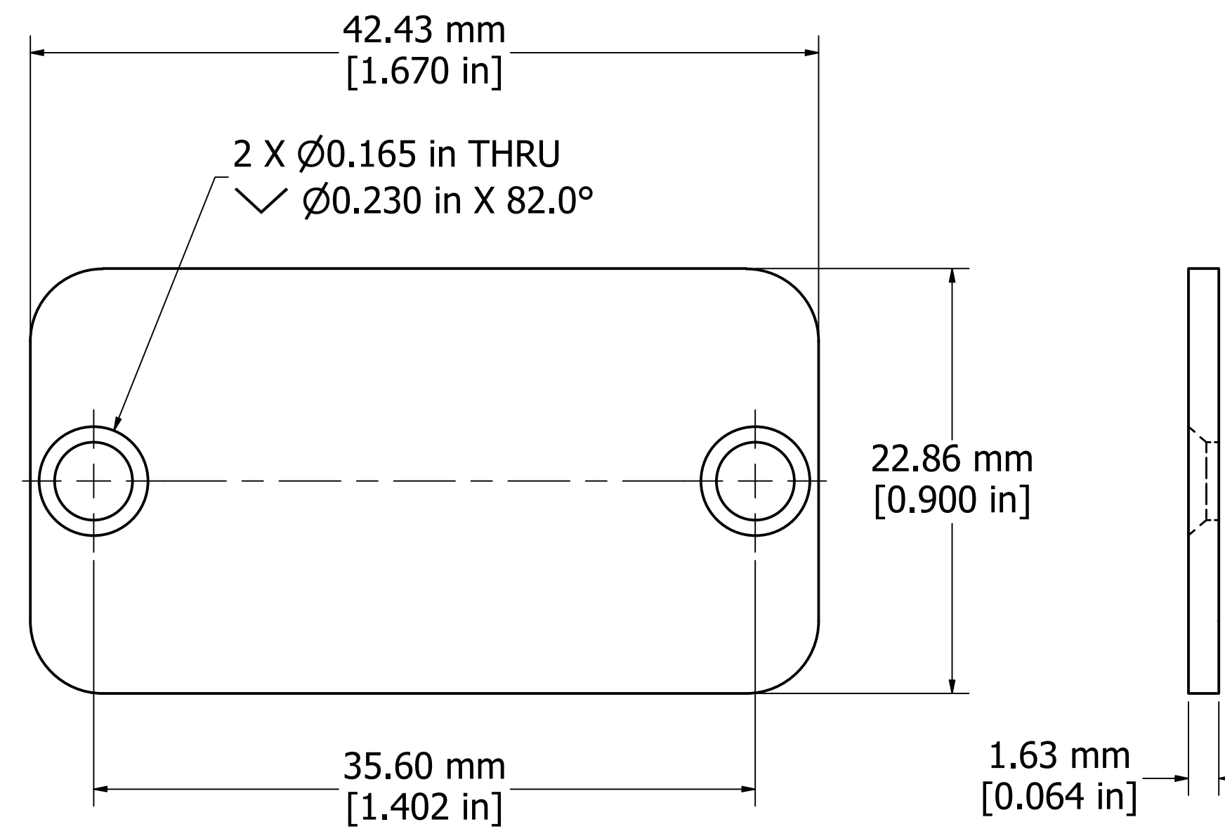
ENDPLATE
