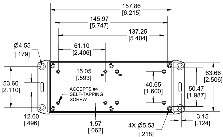
INSIDE LID
